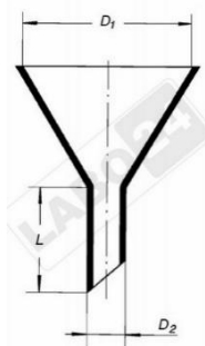
Rys. 4. Lejek laboratoryjny ze szkła borokrzemowego typ 3.3, zwykły kąt 60°, krótka nóżka. (D1/D2/L)
